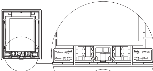
Рис. 1.6. Подключение пульта управления
